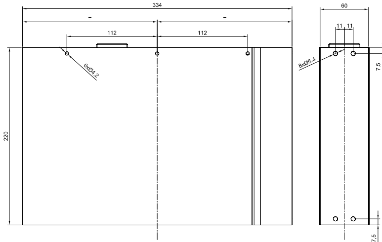
CLMD 33S
