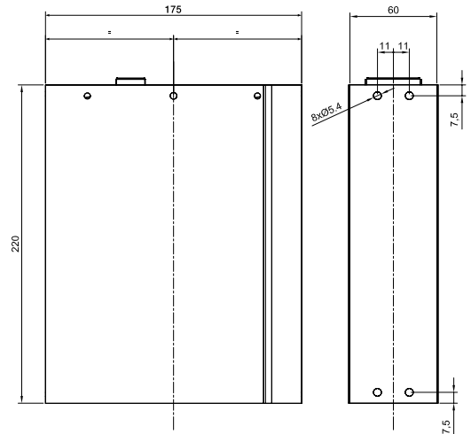
CLMD 13Z
